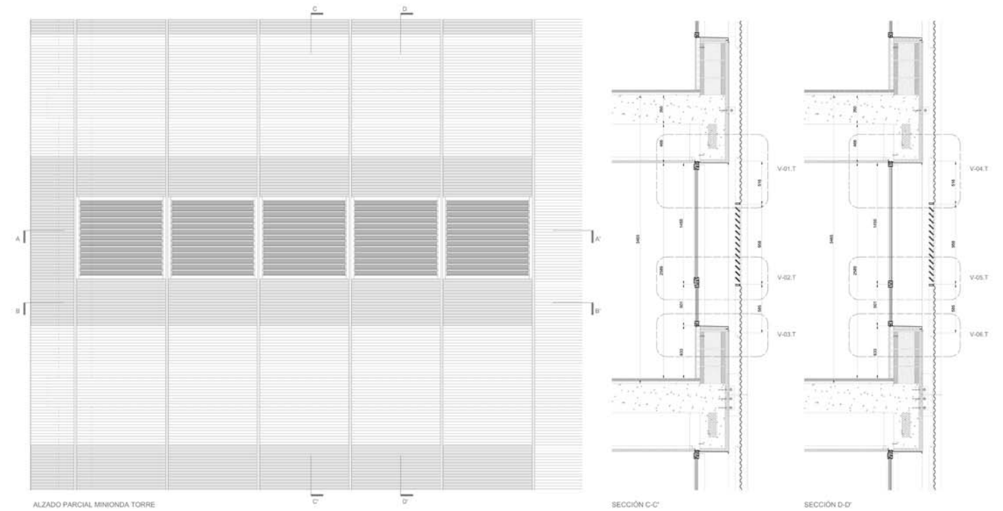
ALZADO PARCIAL MINIONDA TORRE
