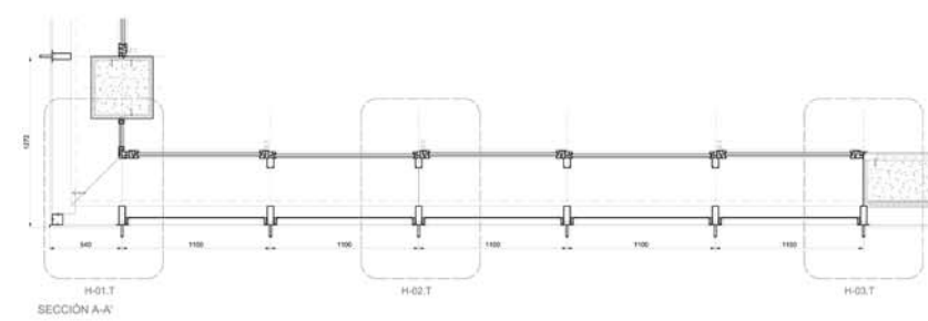
SECCIÓN A-A'
